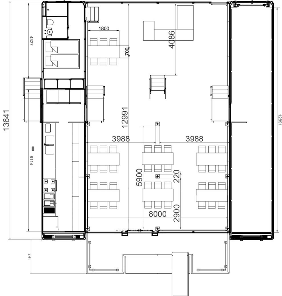
A-A ( 1 : 33 )
