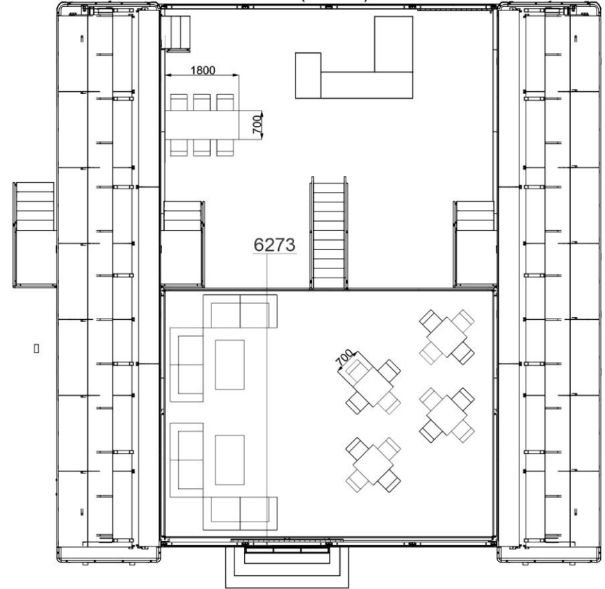
B-B ( 1 : 33 )
