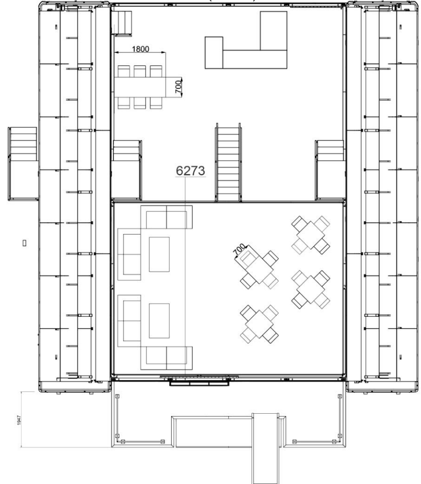
B-B ( 1 : 33 )
